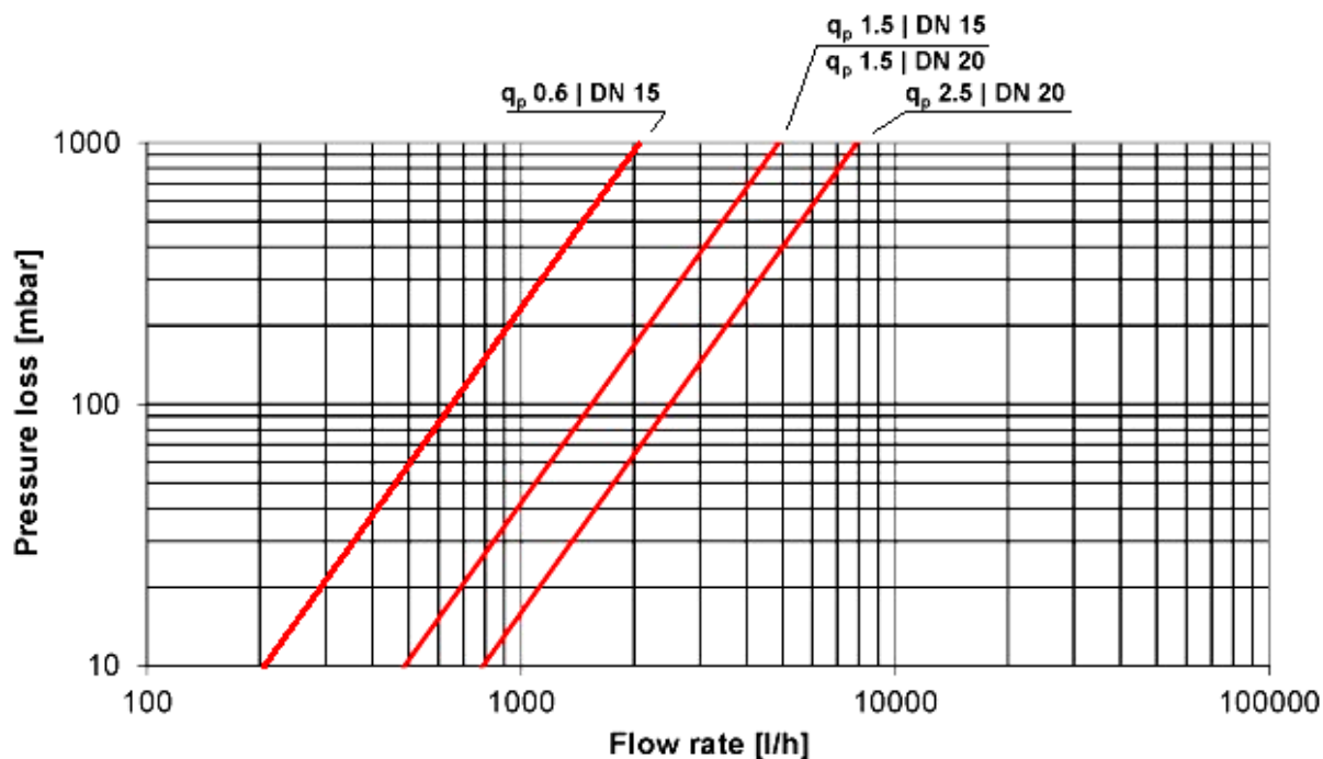
Рисунок 1 - Диаграмма потери давления теплосчетчика SHARKY 774
